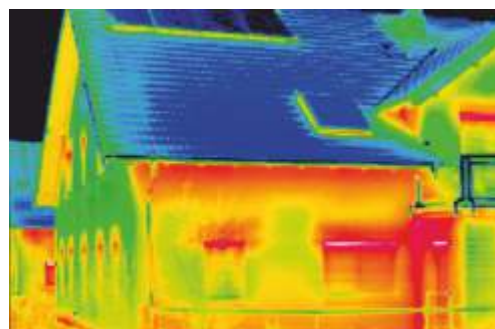
Das Bild zeigt die Untersuchung eines Niedrigenergiehauses auf Fehlstellen in der Isolierung
