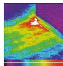
Rohrbruch im Bad vor dem Heizkörper. Ursache: eine defekte Lötstelle.
